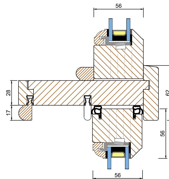
Transom Link D-D (Scale 1:2)
