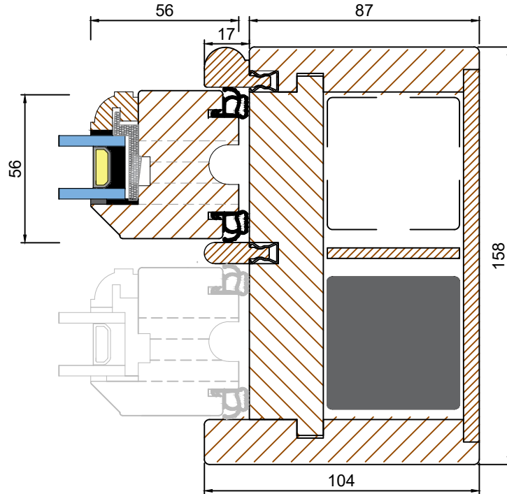
Section C-C - Bottom Sash Jamb
