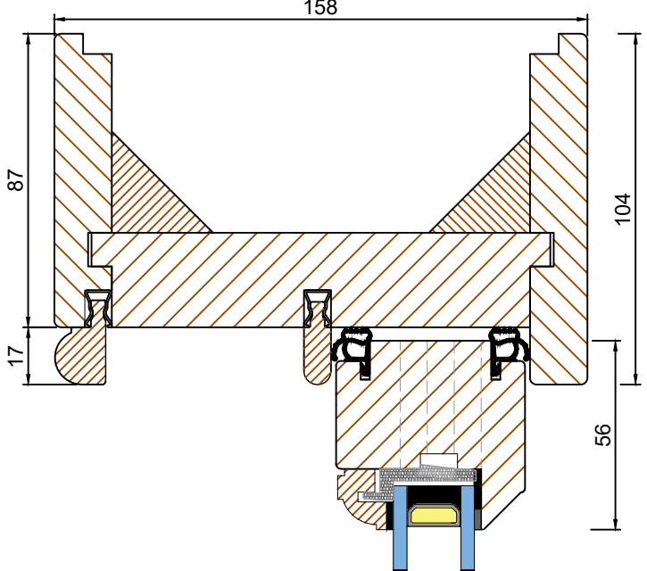
OVOLO BEAD OPTION (Scale 1:2)
