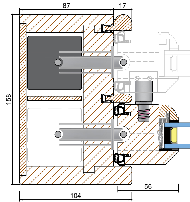
Section A-A - Top Sash Jamb
