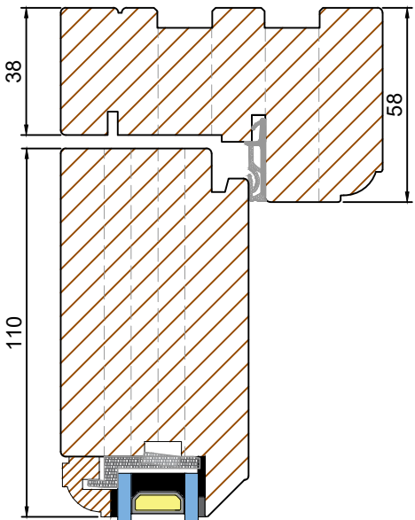
OVOLO BEAD OPTION (Scale 1:2)
