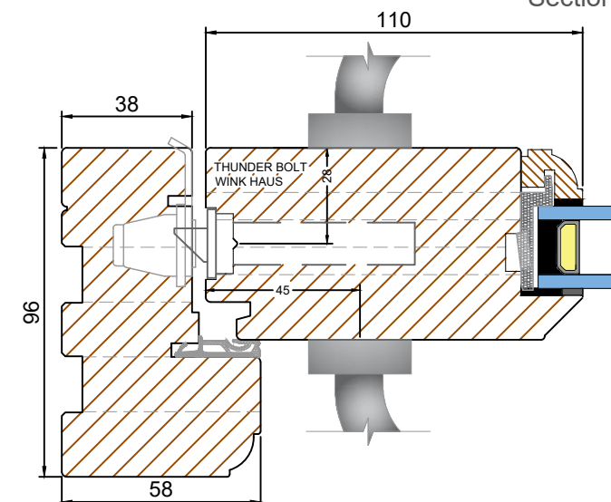
SECTIONS (Scale 1:2) Section D-D - Jamb
