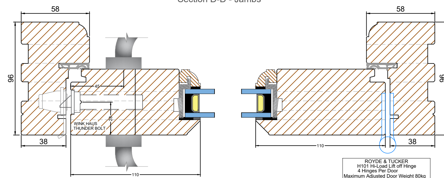
SECTIONS (Scale 1:2) Section D-D - Jamb
