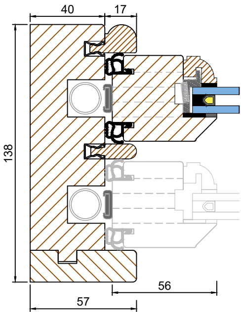
Section C-C - Bottom Sash Jamb
