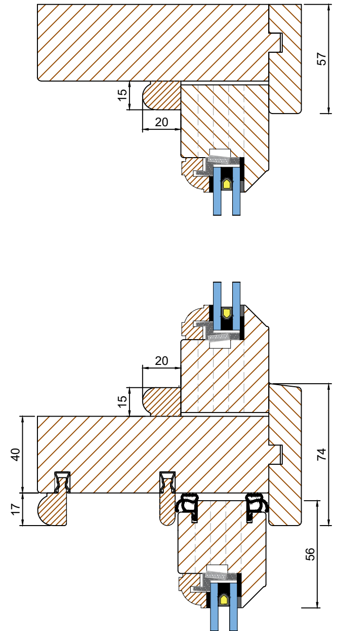
Transom Link D-D (Scale 1:2)
