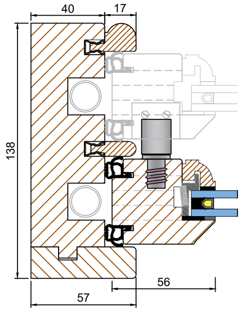
Section A-A - Top Sash Jamb
