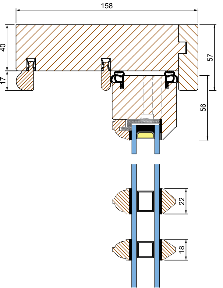
OVOLO BEAD OPTION (Scale 1:2)
